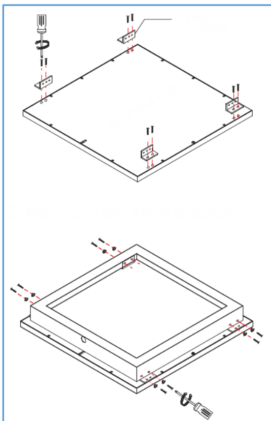
Opbouwrand
