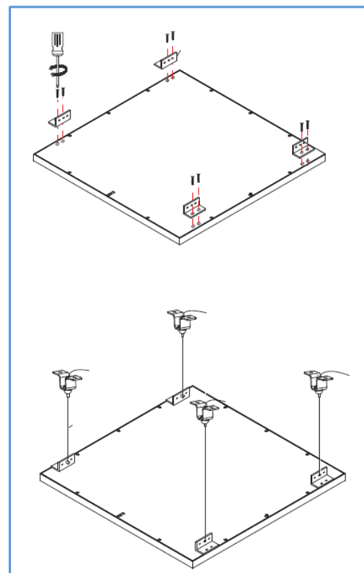
Pendelset
